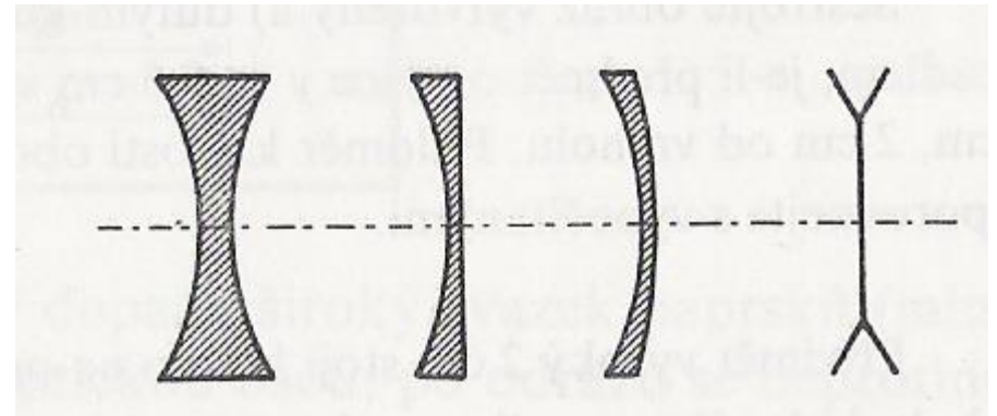
rozptylka
